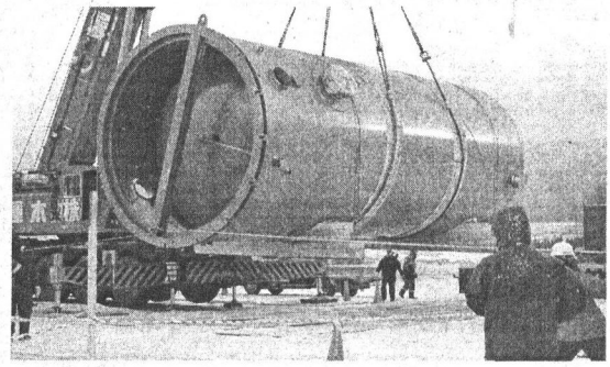
Воздушный ресивер, установленный на заводе СПГ, является пока самым крупногабаритным оборудованием. Его высота – 12 метров, диаметр – 5 метров, вес – почти 50 тонн
